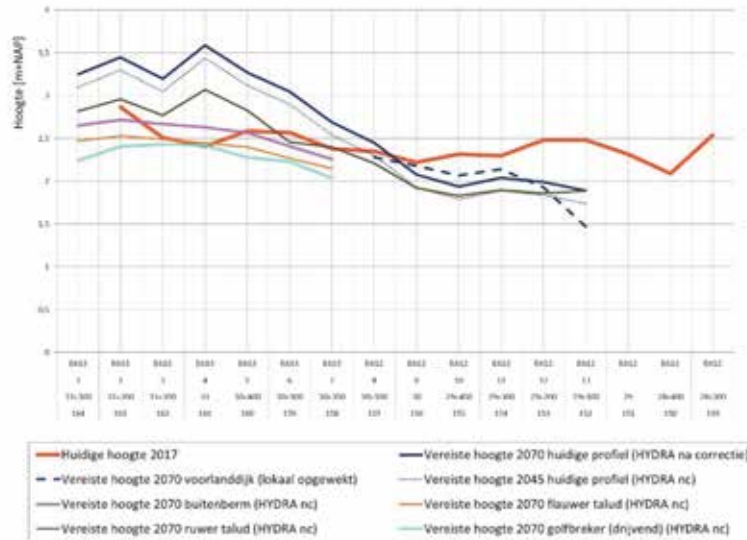
Vereiste dijkhoogte en het effect van diverse maatregelen Uit: Collegebundel dijkversterking Durgerdam November 2018
