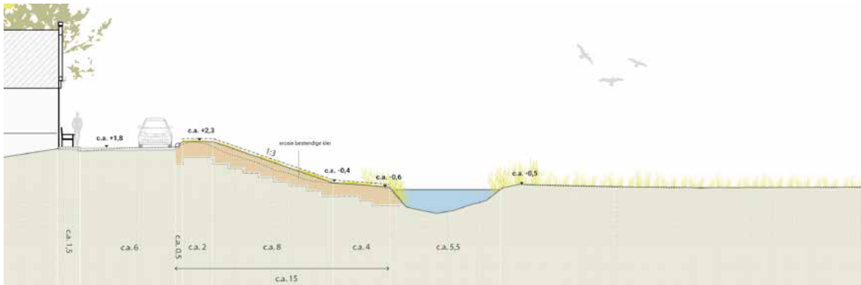
Opbouw profiel IJdoorn: dijkpaal 151
